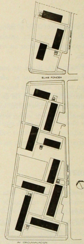
PLANO CONJUNTO
