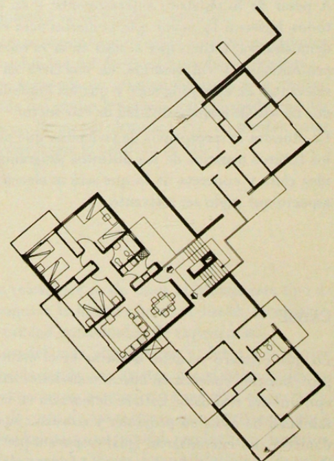
PLANTA DEPTOS TIPO
